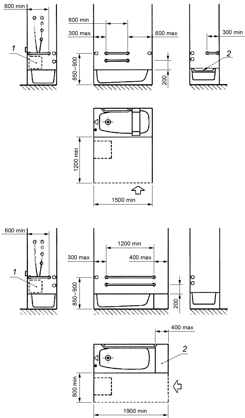
1 - зона размещения органов управления; 2 - сиденье
